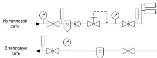
Рисунок 1.5.1 - Схема присоединения потребителей
